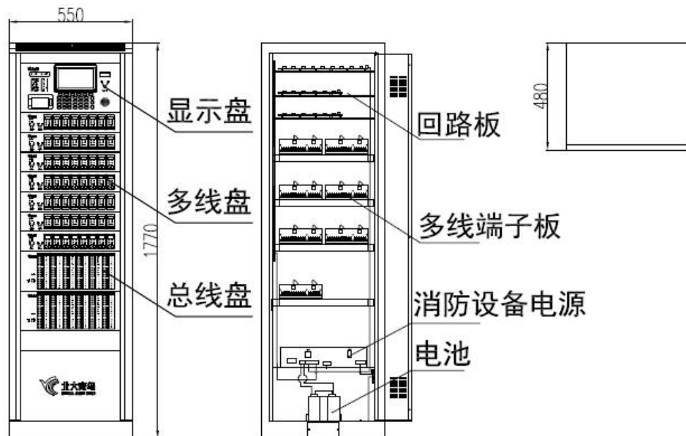
图 2- 1 JB-TG-JBF-11SF 型控制器结构图
