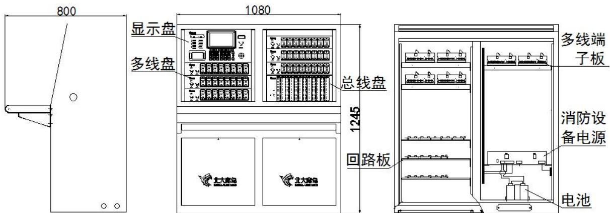
图 2- 3 JB-TG-JBF-11SF 型控制器结构图
